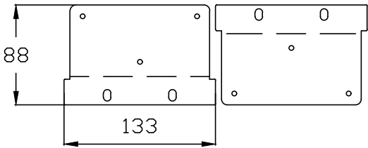
Кронштейн крепления_3U
