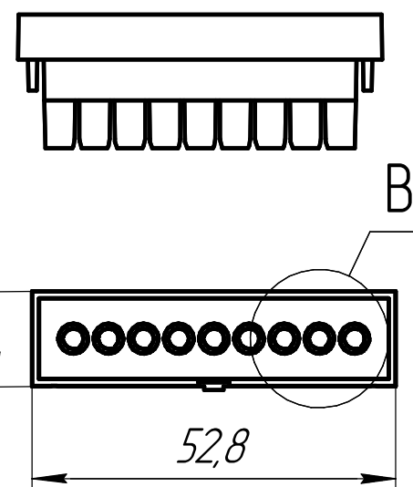
Заглушка, шаг перфорации 5,08мм
