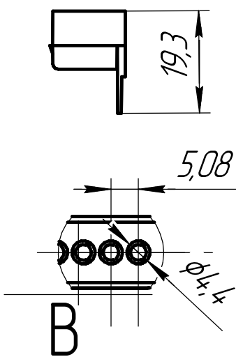
Заглушка, шаг перфорации 5,08мм
