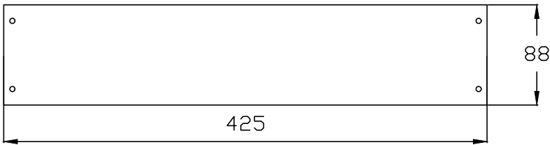
Кронштейн крепления_2U
